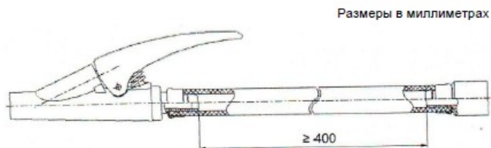
Рисунок 1– Минимальная длина шланга (рукава)
